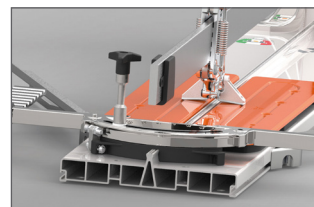
Châssis et support de rail en aluminium
