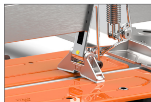
Séparateur de coupe magnétique en aluminium
